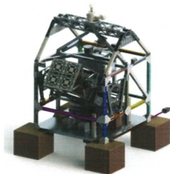
Figura 6: O telescópio imageador de raios X protoMIRAX.
