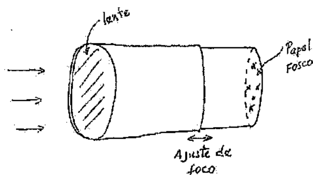
Figura 2.20: Esquema de um telescópio simples. Fonte: autor.
