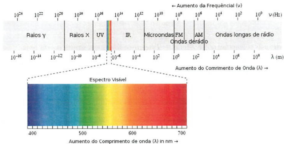
Figura 2.6: O espectro eletromagnético. Note as unidades, 1 \text{ nm} = 0,000000001 \text{ metros} , ou 10^{-9} \text{ m} . Fonte: https://commons.wikimedia.org
