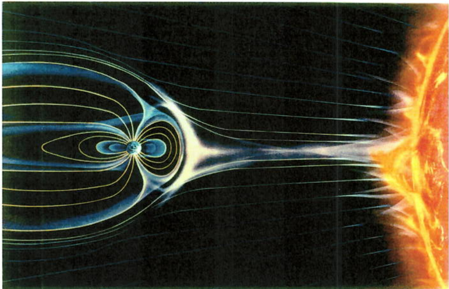
FIGURA 4.24 - VENTO SOLAR E SUA INTERAÇÃO COM A MAGNETOSFERA TERRESTRE. A AÇÃO DO VENTO SOLAR PRESSIONA A MAGNETOSFERA EM DIREÇÃO AO ESPAÇO EXTERIOR.
