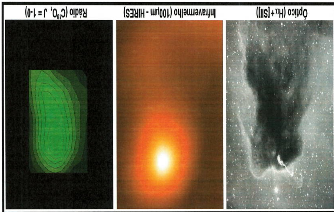
FIGURA 4 – IMAGENS ÓPTICA, INFRAVERMELHO E RÁDIO DO GLÓBULO COMETÁRIO VG33. A IMAGEM ÓPTICA É UMA COMPOSIÇÃO DE IMAGENS OBTIDAS EM H \alpha E SII (REIPUTH, 1997) E A IMAGEM DE RÁDIO É A EMISSÃO DE C ^{18} O (HICKEL E VILAS-BOAS, 2001)
