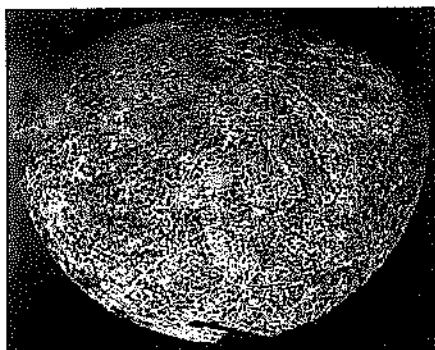
FIGURA 3,5 – MOSAICO DE IMAGENS DO PLANETA MERCÚRIO OBTIDAS COM A Sonda MARINER 10 (NSSDC).
