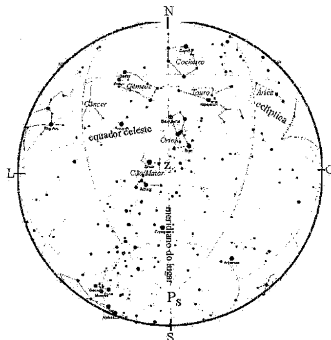
FIGURA 1.11 - PROJEÇÃO DO CÉU PARA SÃO JOSÉ DOS CAMPOS, ÀS 21H, PARA O MEIO DO VERÃO.
