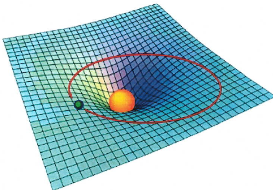
Figura 10.1: Na teoria da Relatividade Geral de Einstein, as massas, principalmente as grandes, causariam deformação no espaço-tempo, de forma semelhante à deformação causada por uma bola de boliche em um colchão de borracha.
