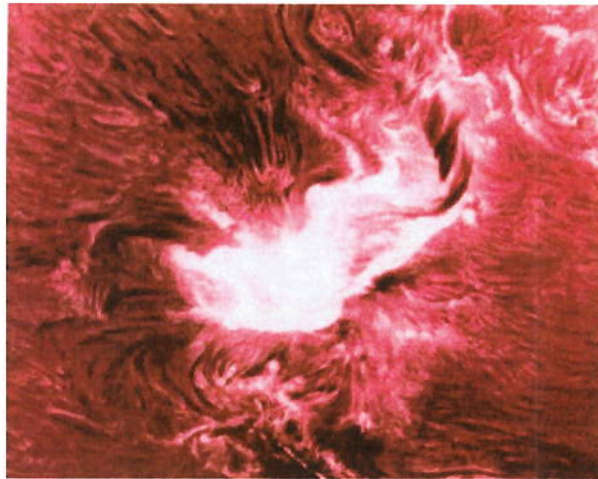
FIGURA 4.21 – EXEMPLO DE “FLARE” SOLAR OBSERVADO NO H-ALFA (FONTE:
