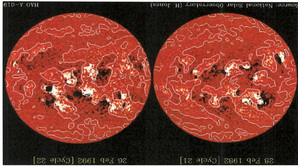
FIGURA 4.16 - (ESQUERDA) POLARIDADES DAS MANCHAS "PRECURSORA" E "SEGUIDORA" DO CAMPO MAGNÉTICO DE REGIÕES ATIVAS NOS HEMISFÉRIOS NORTE E SUL DO SOL DURANTE UM CICLO DE ATIVIDADE. (DIREITA) INVERSÃO DAS POLARIDADES MAGNÉTICAS DAS MANCHAS "PRECURSORA" E "SEGUIDORA" NO CICLO DE ATIVIDADE SEGUINTES (FONTE: NATIONAL SOLAR OBSERVATORY).
