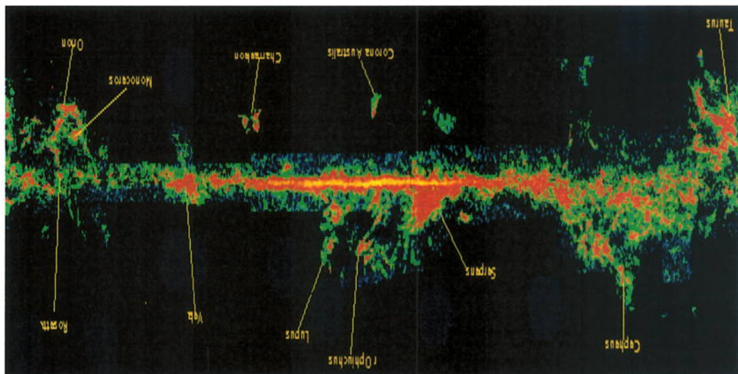
FIGURA 2 – DISTRIBUIÇÃO ESPACIAL DAS NUENS MOLECULARES NA GALÁXIA, DETERMINADA A PARTIR DE CONTAGEM DE ESTRELAS
