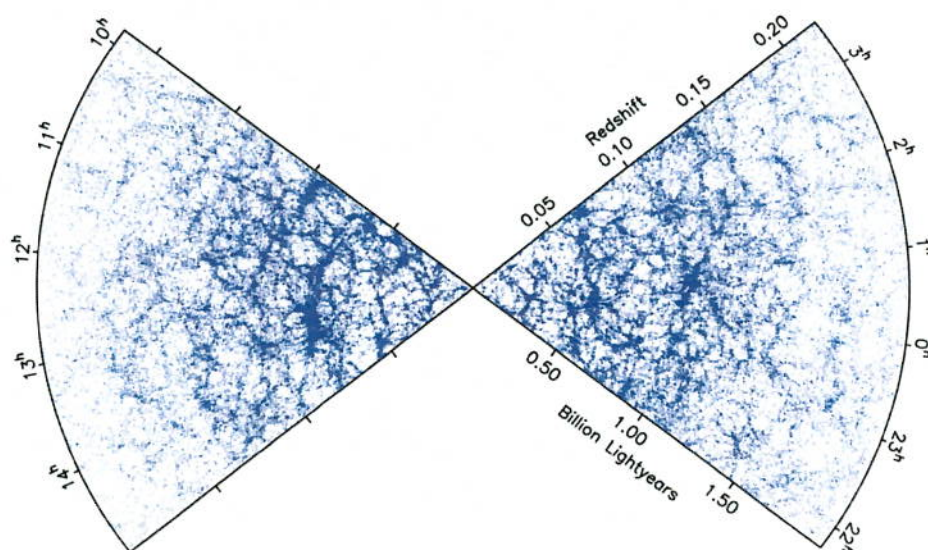
Figura 9.17 – Distribuição das ~ 245.000 galáxias do 2dF. Note-se a presença das estruturas filamentos nos mesmos redshifts observados nos levantamentos anteriores. Fonte: http://www.roe.ac.uk/~jap/2df/
