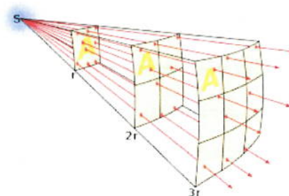
Figura 2.13: A diluição da energia (por unidade de área) com a distância à fonte. De: http://projetosfisicaexperimental.blogspot.com.br/2016/03/leido-inverso-do-quadrado-da-distancia.html
