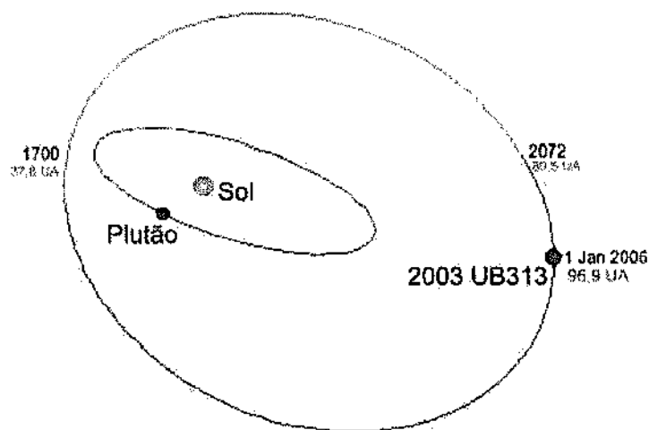
FIGURA 3.15 – ÓRBITA DE ÉRIS (WIKIPEDIA: ÉRIS)
