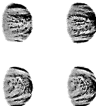
FIGURA 3.6- O PLANETA VÊNUS OBSERVADO PELA SONDA GALILEO (NSSDC).
