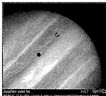
FIGURA 3.10 – IMAGEM DO PLANETA JÚPITER E SEU SATÉLITE IO OBTIDA PELO HUBBLE SPACE TELESCOPE (STSCI).
