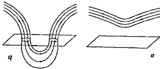
FIGURA 4.14 - EVOLUÇÃO DO CAMPO MAGNÉTICO SOLAR DURANTE O INÍCIO DE UM CICLO DE ATIVIDADE (FONTE: CHOUDHURI, 2007)
