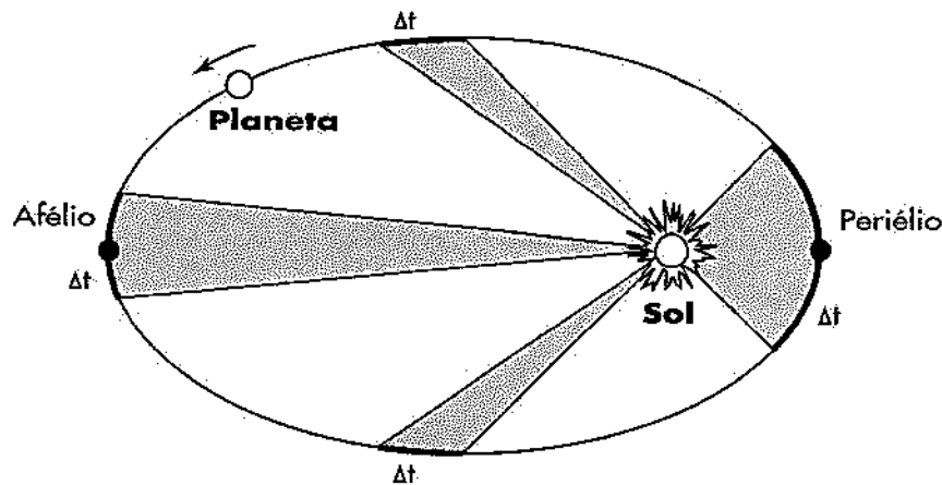
FIGURA 3.3 - LEI DAS ÁREAS.
