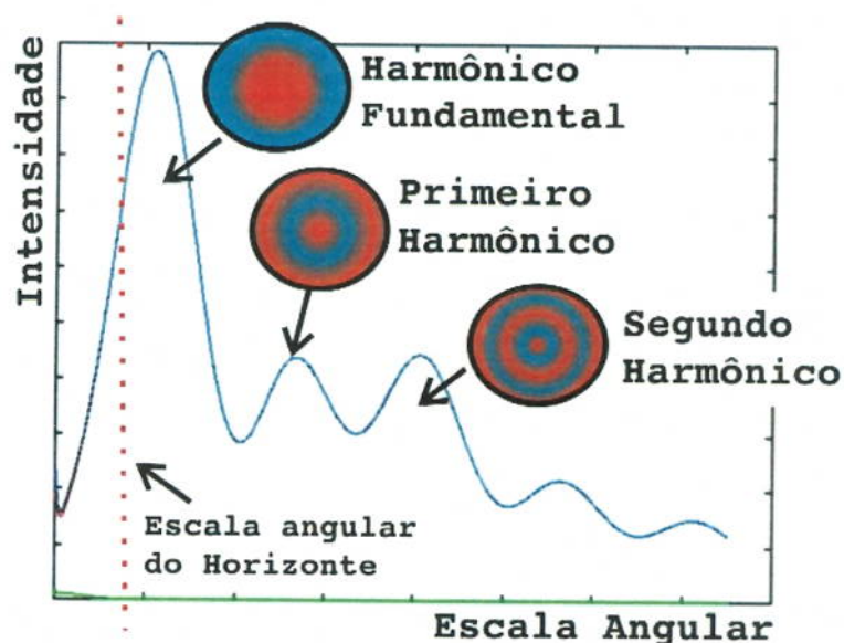
Figura 9.10 – Espectro de potência angular das flutuações de temperatura da RCFM. Em destaque encontram-se os picos acústicos, causados por diferentes processos físicos antes e durante o período da recombinação. Fonte: Autoria própria.
