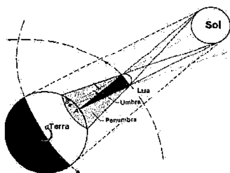
FIGURA 1.20 - ILUSTRAÇÃO DE UM ECLIPSE TOTAL DO SOL (FORA DE ESCALA) COM FOTOGRAFIA FEITA A PARTIR DO PONTO B DONDE É AVISTADO COMO PARCIAL (FOTO DE ANDRÉ MILONE, NO OBSERVATÓRIO DO VALONGO/UFRJ, RIO DE JANEIRO, 1987).
