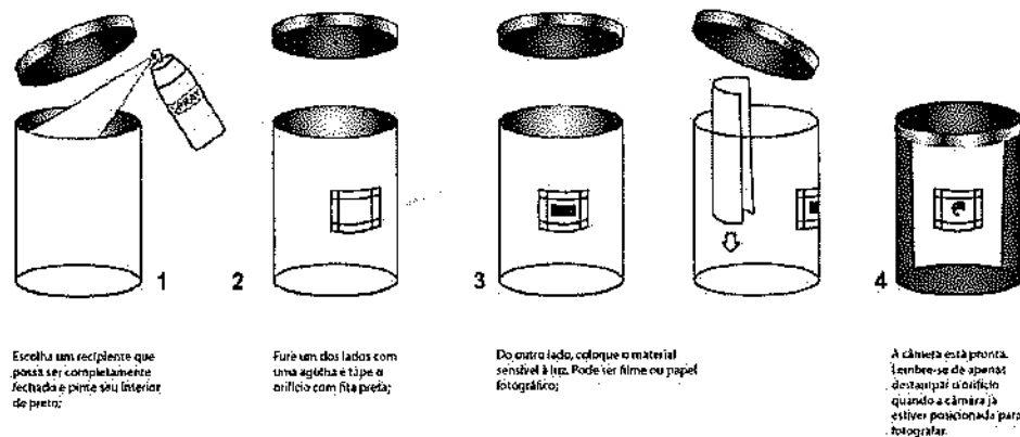
Figura 2.18: Passo a passo de como construir uma câmara pinhole. Obtida em https://www.jornalufgonline.ufg.br/n/30640-camera-pinhole .
