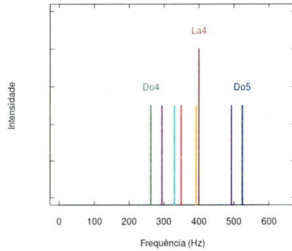
Figura 2.2: O espectro acústico de um piano na 4ª oitava.
