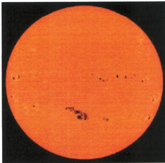
FIGURA 4.6 - DISCO SOLAR COM MANCHAS SOLARES. (FONTE:
