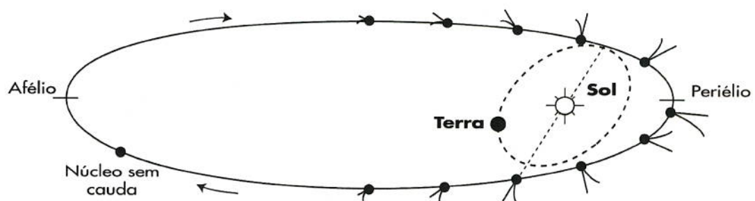
FIGURA 3.17 - UM EXEMPLO DE ÓRBITA DE COMETA.
