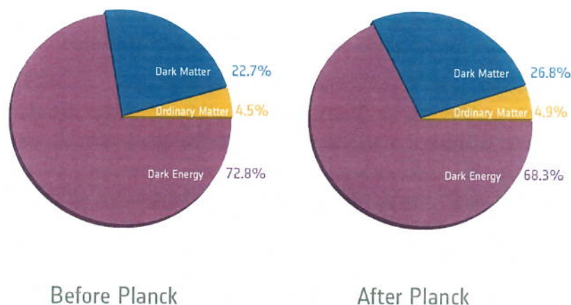
Figura 9.23– Distribuição percentual dos componentes de matéria e energia no Universo.
