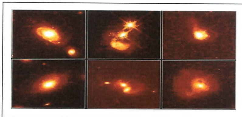
Figura 8.16 – Regiões hospedeiras de quasares.
