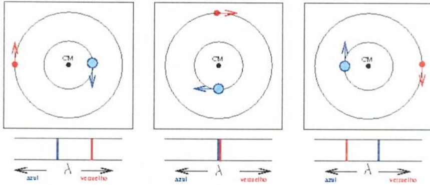
Figura 2.10: Um sistema binário com a representação do deslocamento Doppler da linha espectral de um mesmo elemento à medida que as estrelas se movem em órbita. Fonte: http://astro.ifurgs.br/bin/binarias.htm .
