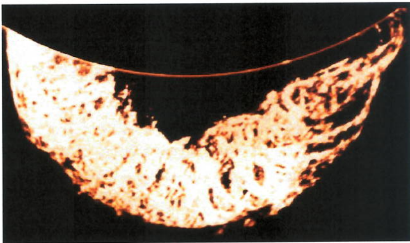
FIGURA 4.11 - PROEMINÊNCIA SOLAR OBSERVADA EM H-ALFA. (FONTE: http://science.msfc.nasa.gov/ssl )
