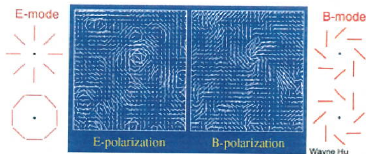
Figura 9.12 – O padrão gradiente (escalar) é chamado de modo E (E-mode) no jargão dos pesquisadores da RCFM. O padrão escalar é simétrico, refletindo as condições físicas que o geraram (espalhamento Thomson). O padrão rotacional (tensorial) indica uma distorção da radiação devido à interação com objetos massivos pelos quais ela passou (ou pela altíssima densidade do Universo primordial, onde ela também pode ter sido gerada), permitindo o mapeamento da distribuição de matéria ao longo do caminho ótico da RCFM. Fonte: Wayne Hu (2001).
