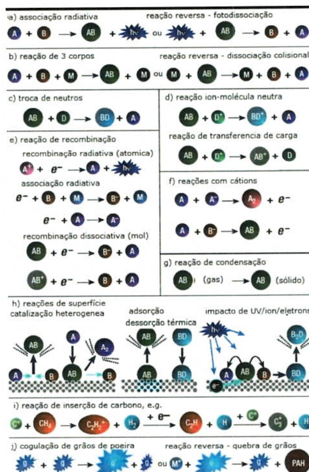
Figura 11. 2 - Representação esquemática das principais reações químicas que ocorrem nas nuvens interestelares. O símbolo PAH corresponde a Hidrocarbonetos Poli Aromáticos (Adaptado de Fraser (2002)).
