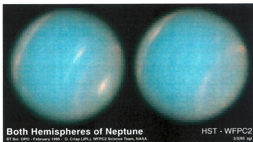
FIGURA 3.13 – IMAGENS DOS DOIS HEMISFÉRIOS DO PLANETA NETUNO OBTIDAS COM O HUBBLE SPACE TELESCOPE (STScI).
