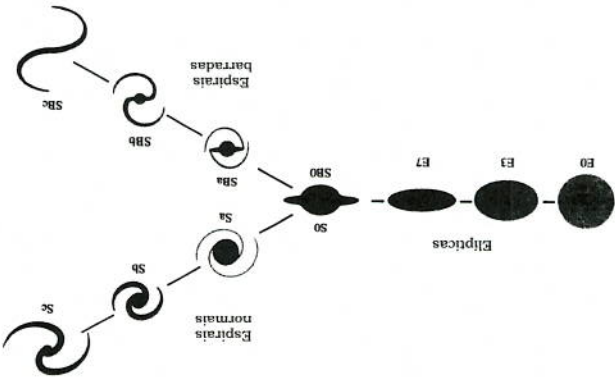
Figura 8.7 – Galáxias espirais Sa, Sb e Sc, com a clara variação na forma e estrutura dos braços. Note-se a ausência, nessa foto, de espirais com barra.
