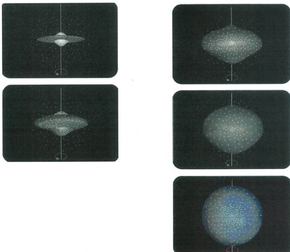
Figura 8.11 – De cima para baixo, vemos uma nuvem de gás em expansão; no centro a nuvem começa a colapsar sob o efeito da matéria concentrada no seu interior. Embaixo, estrelas de população II são formadas no núcleo. As regiões externas do globo caem para o centro e criam um disco de gás em rotação onde estrelas de população I irão, futuramente, se formar (Ref. Adaptada de Seeds, 2000)
