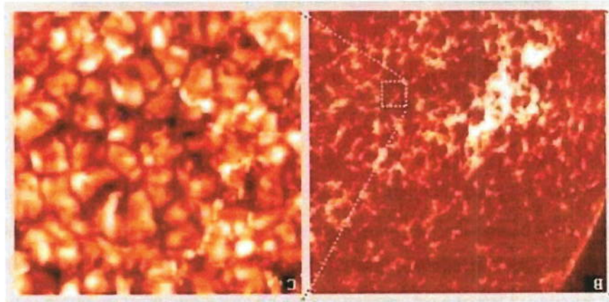
FIGURA 4.3 - IMAGENS MOSTRANDO O FENÔMENO DE GRANULAÇÃO DA FOTOSFERA SOLAR. (FONTE: HTTP://ASTRO.IFE.UFRGS.BR/ESOL/ESOL.HTM .)
