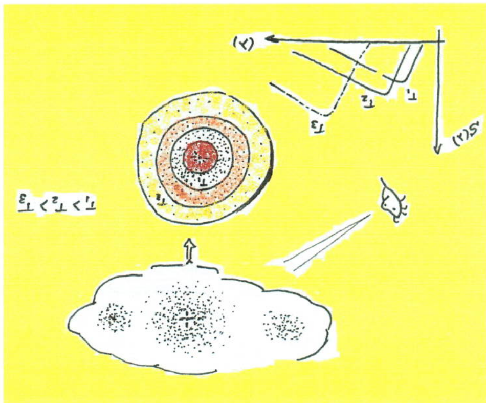
FIGURA 3 – REPRESENTAÇÃO ESQUEMÁTICA DO AQUECIMENTO DA REGIÃO CENTRAL DE UM GLÓBULO POR UMA ESTRELA EM SEUS ESTÁGIOS PRIMORDIAIS.
