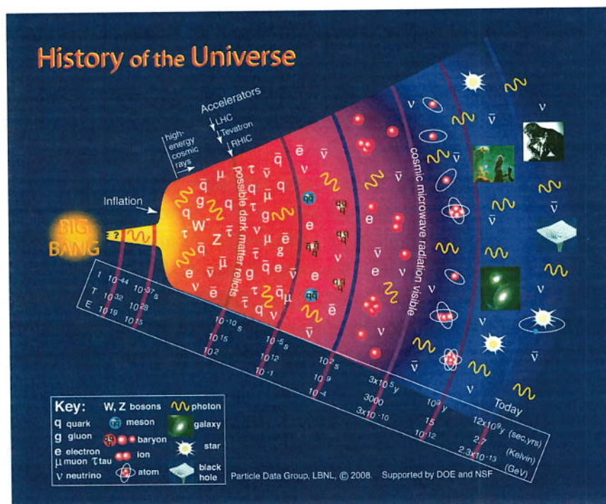
Figura 9.6 – Diagrama descritivo da história do Universo. Os números na parte inferior descrevem, respectivamente, o tempo (época) e a energia (temperatura) correspondentes a cada evento. Cada linha magenta representa um grande evento na história cósmica. Da esquerda para a direita: época da Grande Unificação ( 10^{-44} s); inflação ( 10^{-32} s); desacoplamento das forças eletrofraca e forte ( 10^{-10} s); nucleossíntese primordial (entre 10^{-2} s e 180 s); desacoplamento matéria-radiação ( 3 \times 10^5 anos); formação de estruturas ( 1 \times 10^9 anos); época atual ( 12 \times 10^9 anos). Fonte: Particle Data Group, LBNL (2008).
