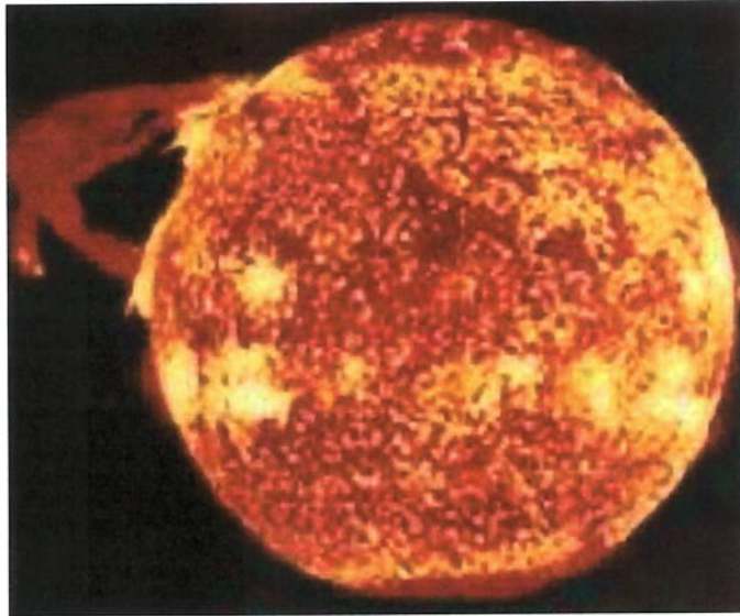
FIGURA 4.12 - IMAGEM EM RAIOS-X DO SOL, ORTIDA PELO SATÉLITE SKYLAB EM 19 DE DEZEMBRO DE 1973. É MOSTRADA UMA DAS MAIS IMPRESSIONANTES PROEMINÊNCIAS JÁ REGISTRADAS. (FONTE: LABORATORIO ESPACIAL SKYLAB - NASA).
