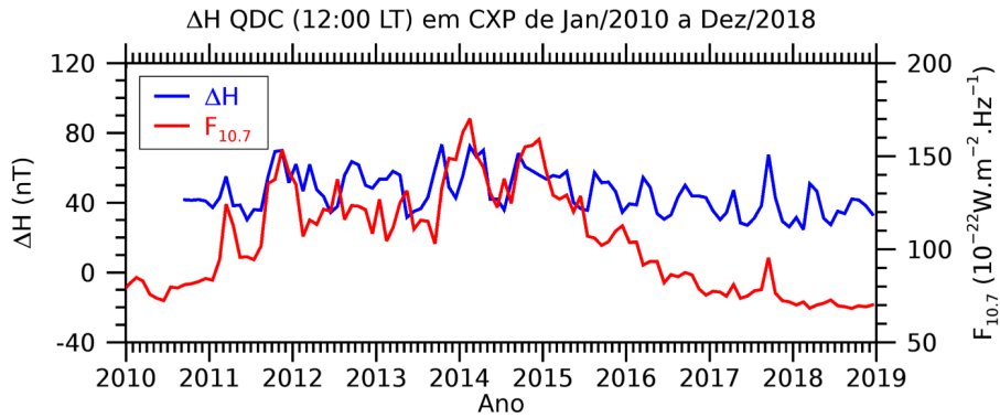
Figura 6.6 - Série temporal da amplitude da \Delta H_{QDC}(12:00LT) da estação de Cachoeira Paulista e o respectivo valor do F_{10.7} mensal entre os meses de janeiro de 2010 e dezembro de 2018.
