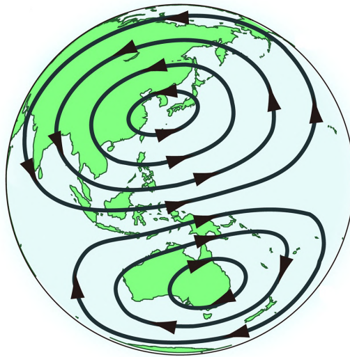
Figura 3.4 - Representação esquemática padrão diurno dos sistemas de correntes Sq.
