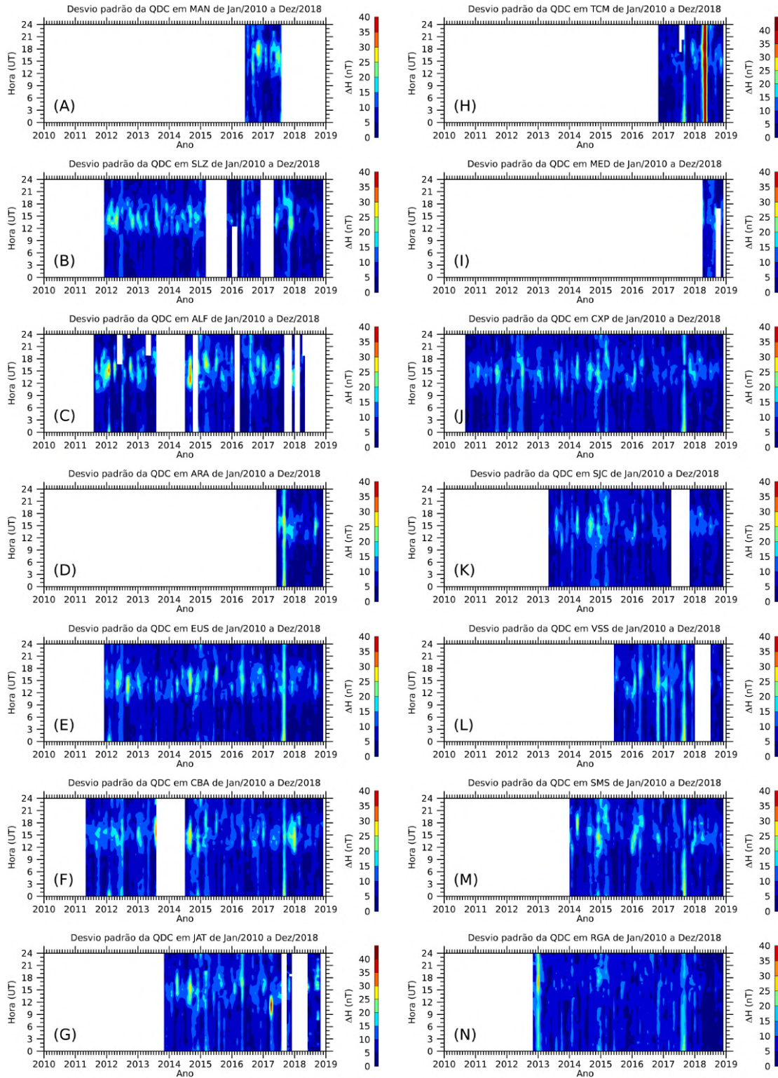
Figura 6.16 - Desvio padrão das QDCs mensais da componente horizontal do campo geomagnético, obtido a partir dos dados das estações magnéticas da Embrace MagNet entre janeiro de 2010 e dezembro de 2018.
