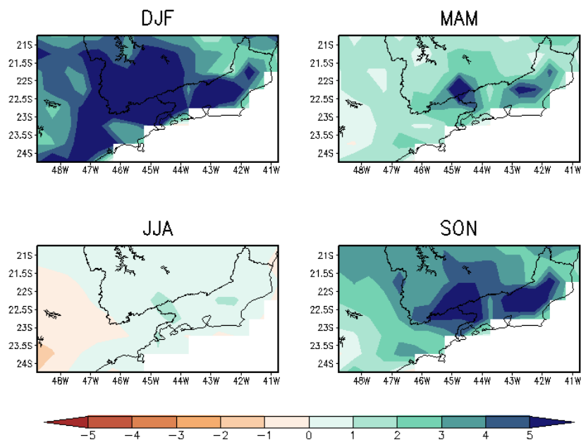
Figura 13: Viés de precipitação ( \text{mm}\cdot\text{dia}^{-1} ) para a simulação Reg5km e para o período de 2005 a 2015, valores negativos, cores laranjas, (positivos, cores verdes) representam viés negativo (positiva). As siglas idem figura 2.
