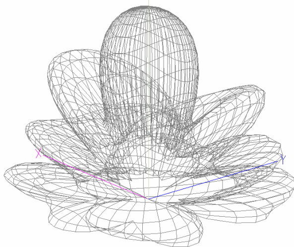
Fig. 5.36 – Diagrama de irradiação tridimensional da antena dipolo similar à do sistema LOFAR para a frequência de 90 MHz.
