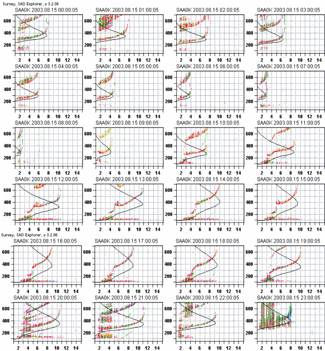
Figura 3.10 - Série de ionogramas obtidos no dia 15 de agosto de 2003 no sítio de São Luís – MA.
