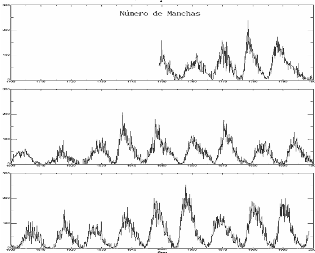
Figura 1.8- Ciclo das manchas solares
