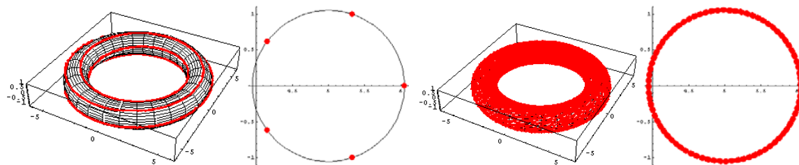
Figura 3: Diferença entre comportamento periódico e quase-periódico no espaço de estados e no Mapa de Círculo
