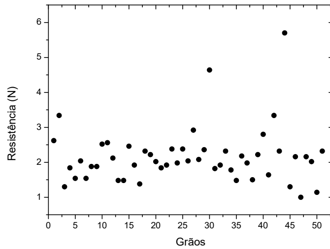
Figura 12 - Dispersão das forças de ruptura razão 0,80
