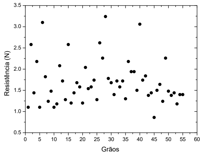
Figura 15 - Dispersão das forças de ruptura razão 0,95
