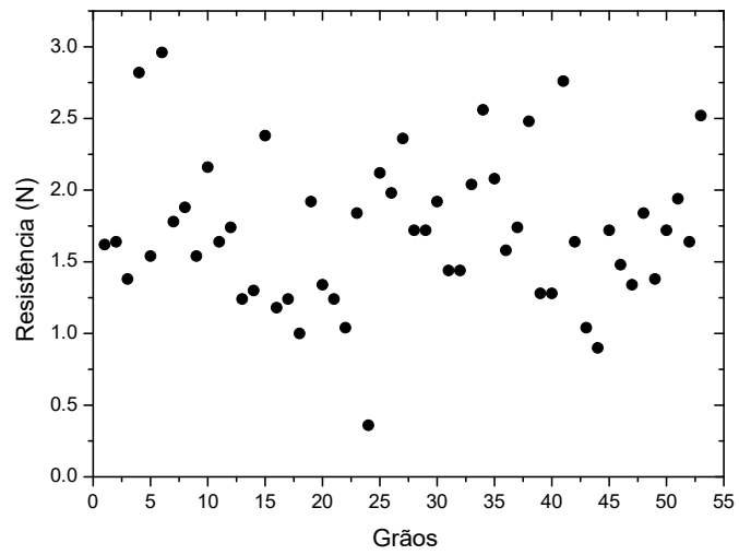
Figura 14 - Dispersão das forças de ruptura razão 0,90
