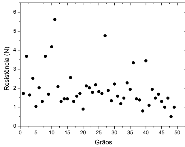
Figura 13 - Dispersão das forças de ruptura razão 0,85
