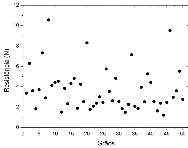
Figura 10 - Dispersão das forças de ruptura razão 0,60
