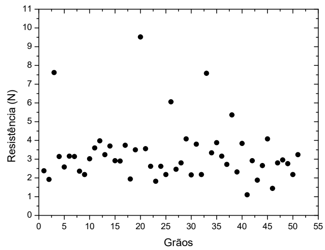
Figura 11 - Dispersão das forças de ruptura razão 0,70
