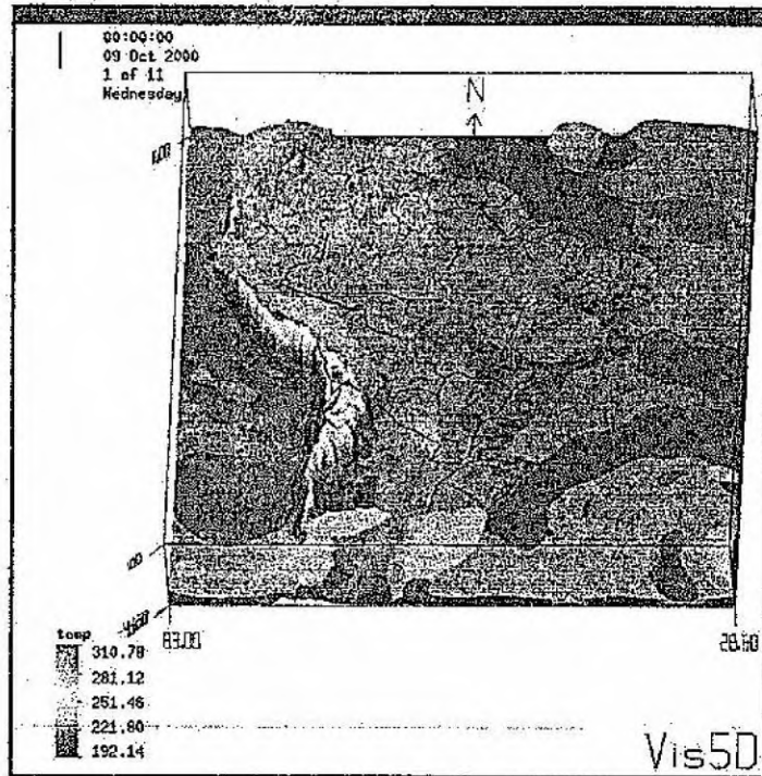
Fig.3 – Visualização de variável temperatura pelo Vis5D
